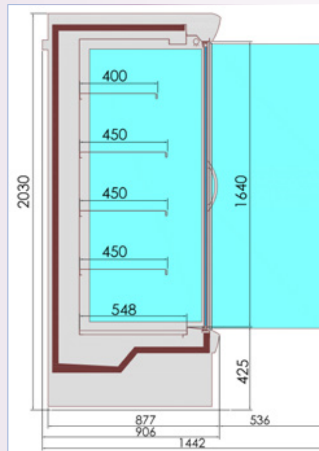
Coupe ZEUS porte ouverte
