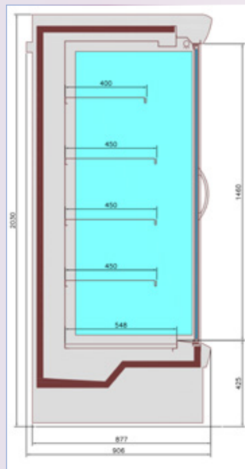
Coupe ZEUS porte fermée
