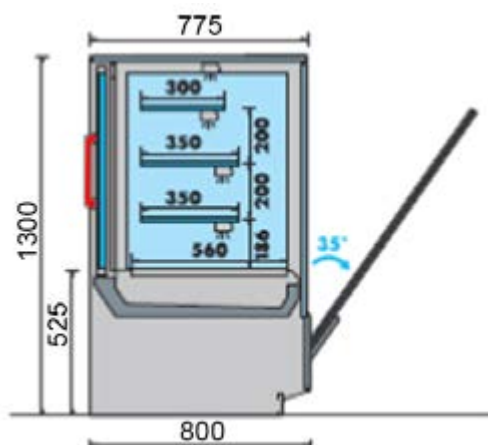
Version vitre rabattable à l'avant L.700 portes battantes à l'arrière
