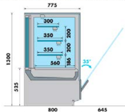
Version vitre rabattable à l'avant L.1000-1250-1500 portes coulissantes à l'arrière
