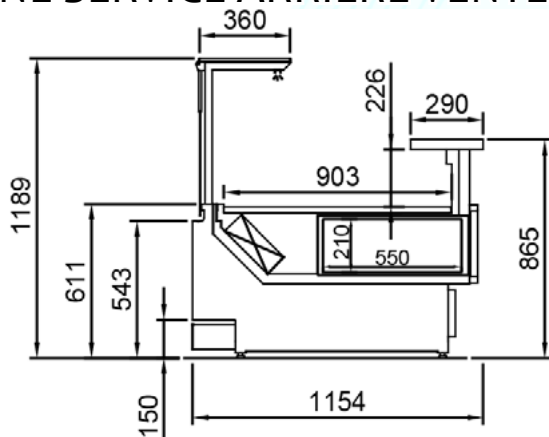
MOKA C3 : Version ventilé avec réserve
