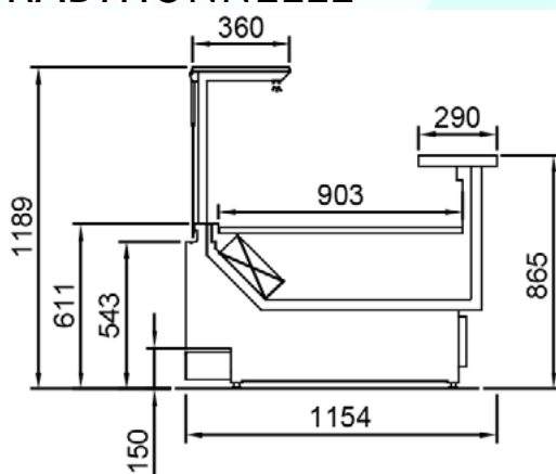
MOKA V3 : Version ventilé sans réserve
