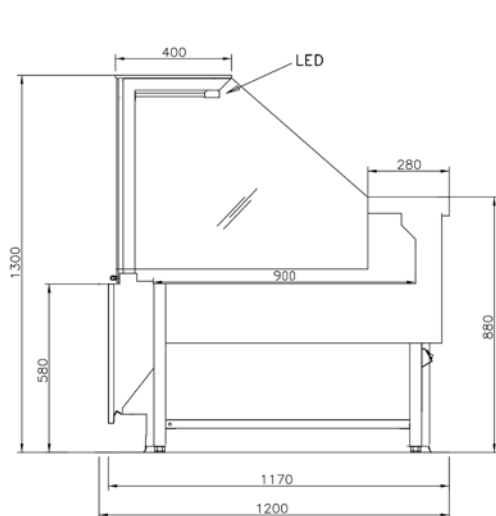
Version standard réfrigérée ventilée
