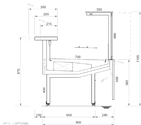
Version réfrigérée ventilé - cuve étroite 700 ouverture à la française
