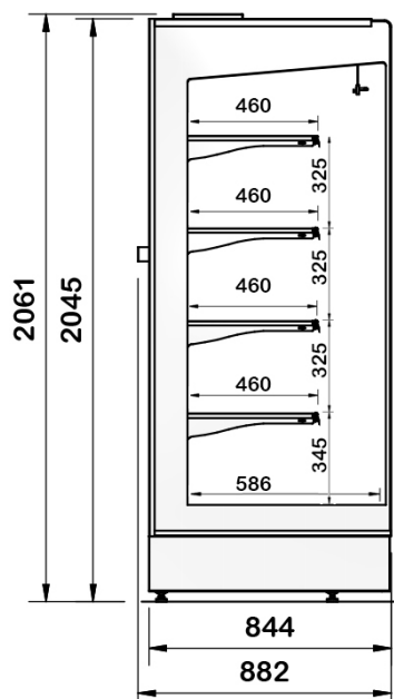
Version standard 4 niveaux d'étagères
