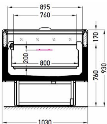
Version avec couvercle
