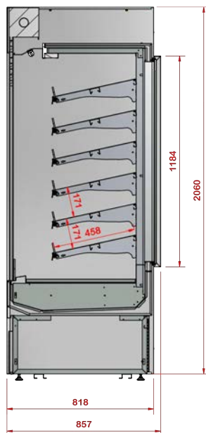
Version chargement arrière sans portes avant
