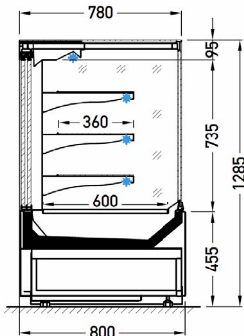
Version porte arrière coulissante
