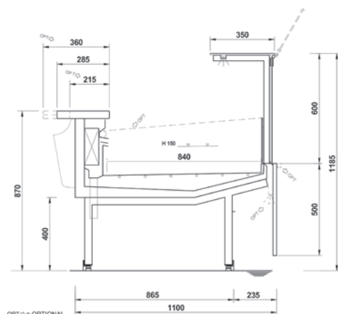
Version froid statique ou bi-dynamique Vitre relevable
