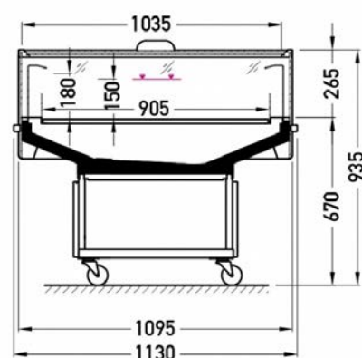
Version avec couvercle coulissant
