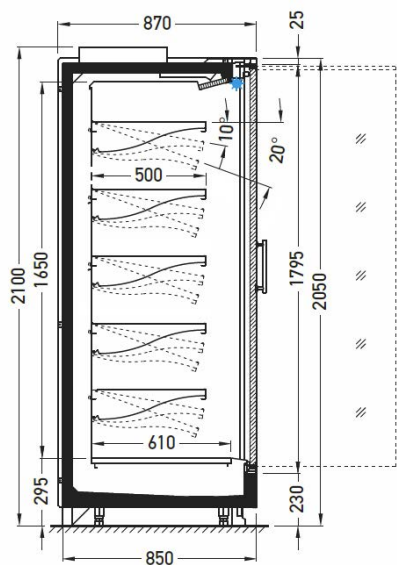
Versions à portes battantes 850 - 2000 - 5 niveaux
