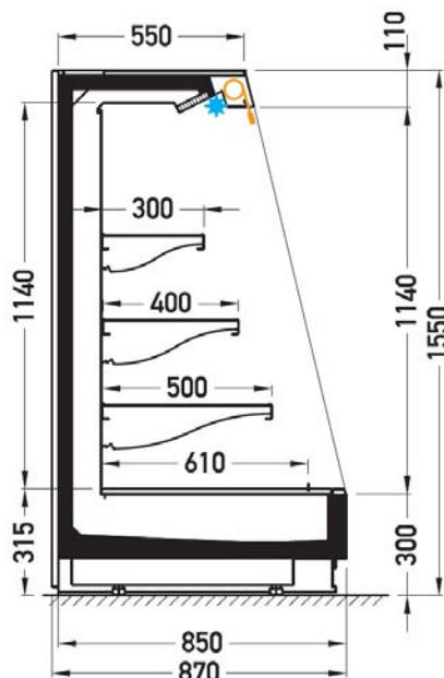
Version sans porte
