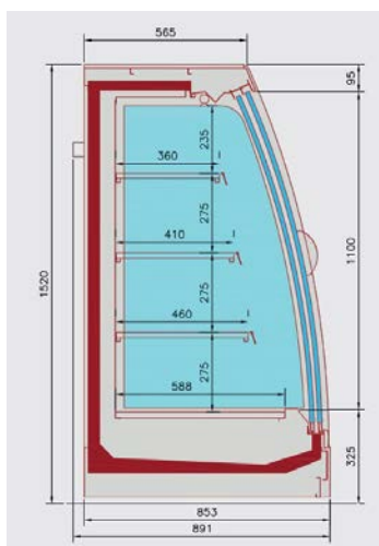
PRAGUE 850 BOMBÉE COULISSANTES
