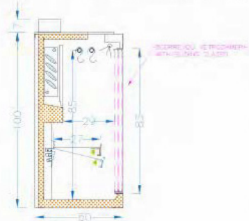
Version un niveau fermeture coulissante double vitrage
