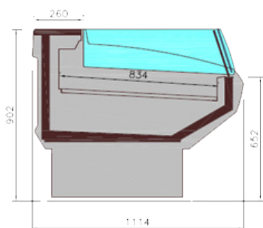
LS standard sans réserve
