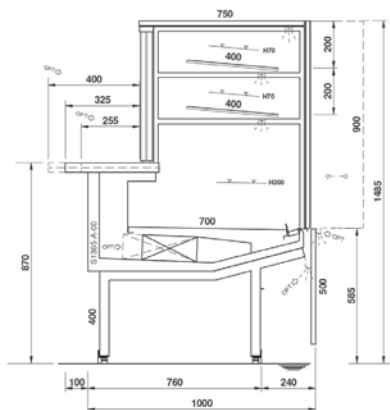
Tour 1500 - 2 niveaux d'étagères Canalisable avec P. 800 mm
