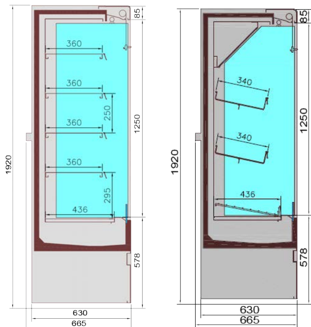
Version standard inox ou peinte
