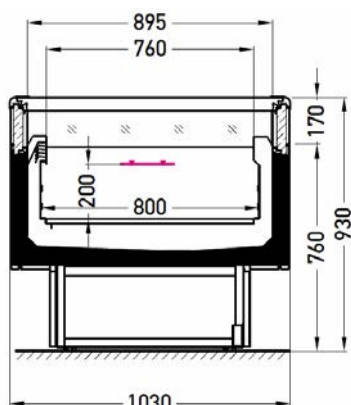
Version sans couvercle
