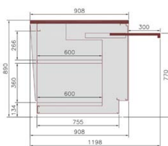
Caisse PMR tablette couissante
