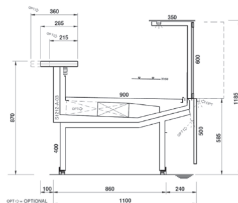
Version réfrigérée ventilé - cuve 900 ouverture à la française
