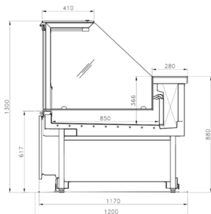
Version réfrigérée statique-ventilée
