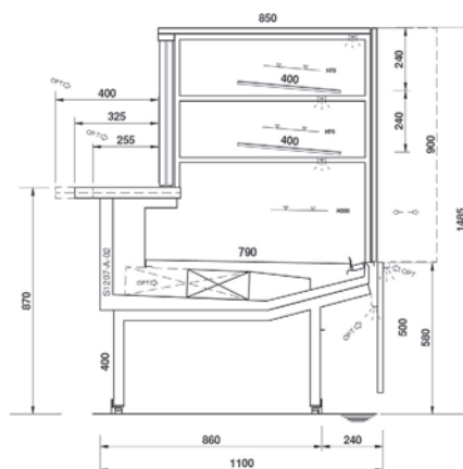
Tour 1500 - 2 niveaux d'étagères Canalisable avec P. 900 mm
