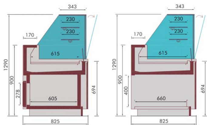
Version avec réserve
