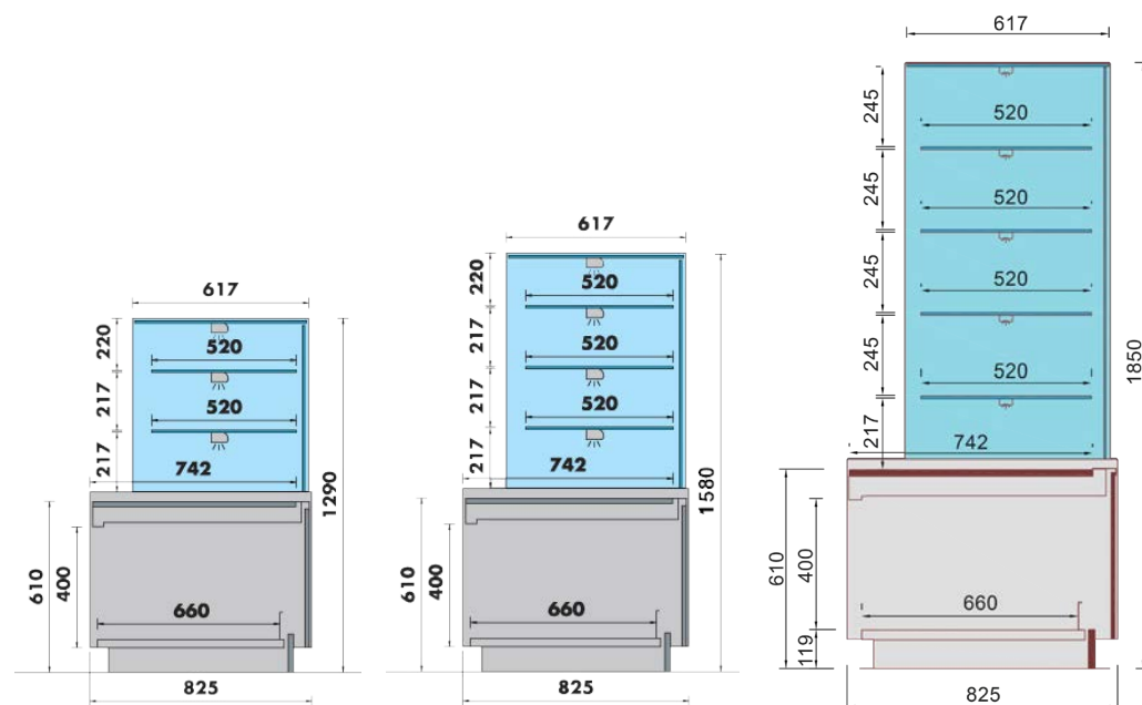
Tour viennoiserie STANDARD
