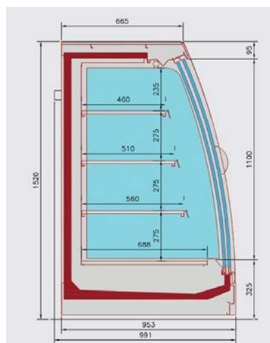
PRAGUE 950 BOMBÉE COULISSANTES
