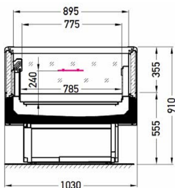
Version sans couvercle
