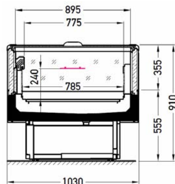
Version avec couvercle coulissant
