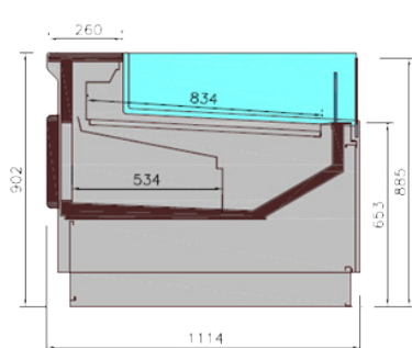
LS standard avec réserve
