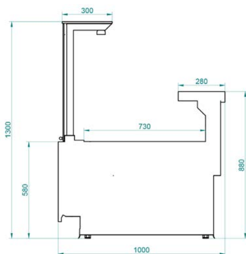
Version SLIM réfrigérée ventilée
