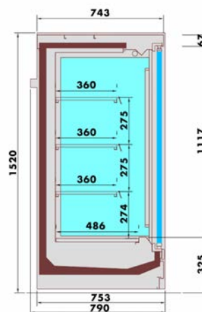
PRAGUE 750 DROITE BATTANTES
