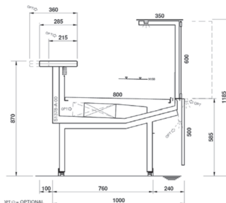
Version réfrigérée ventilé - cuve 800 ouverture à la française
