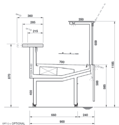
Version réfrigérée ventilé cuve étroite 700 vitre relevable
