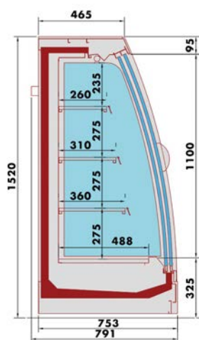
PRAGUE 750 BOMBÉE COULISSANTES
