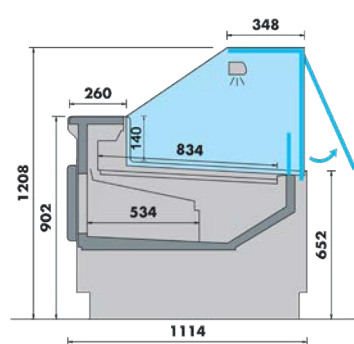
Avec réserve réfrigérée
