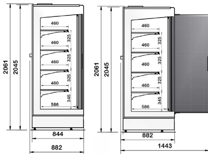
Version à portes COUPE porte fermée
