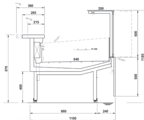
Version froid statique ou bi-dynamique Vitre ouverture à la française
