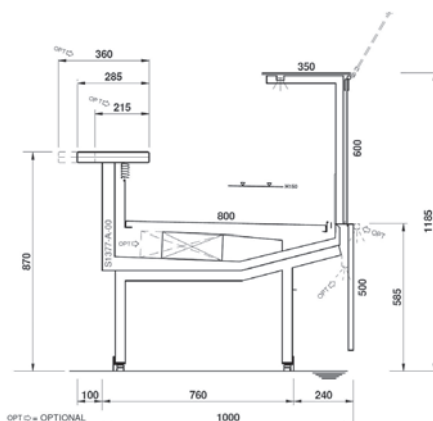
Version réfrigérée ventilé cuve 800 vitre relevable
