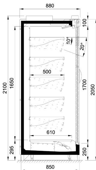
Versions à portes coulissantes 850 - 2000 - 5 niveaux
