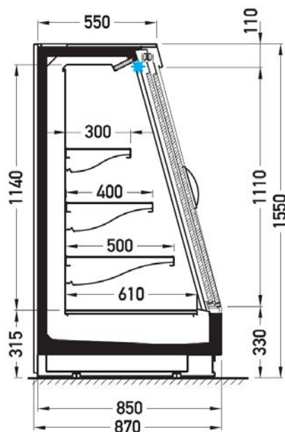
Version avec porte droite oblique
