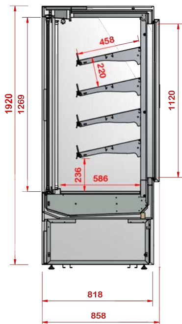
Version chargement arrière avec portes avant battante ou coulissante
