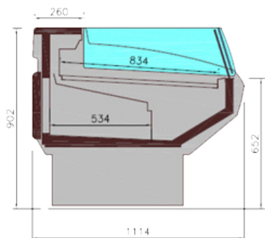
LS standard avec réserve réfrigérée
