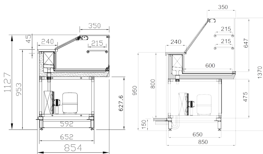
Version vitre basse
