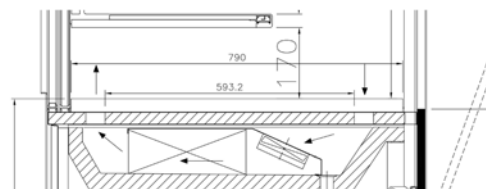
Coupe plateau d'exposition
