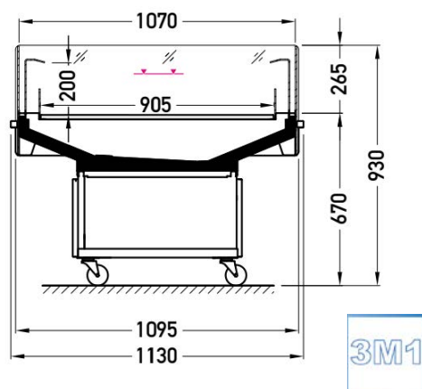
Version sans couvercle
