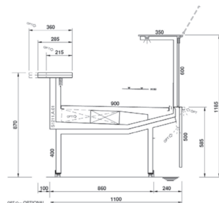
Version réfrigérée ventilé cuve 900 vitre relevable
