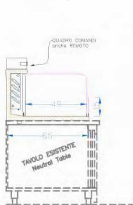
Version à poser
