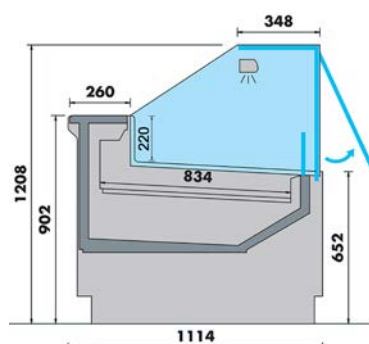
Sans réserve réfrigérée
