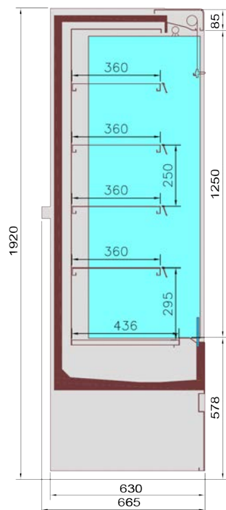
Version standard inox ou peinte
