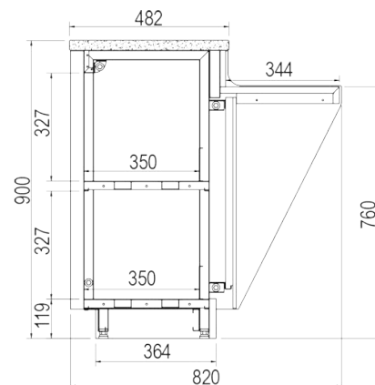
Caisse PMR tablette fixe
