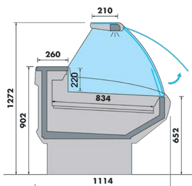
Sans réserve réfrigérée
