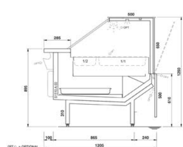
Détail bain marie L.938
