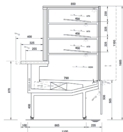
Tour 1700 - 3 niveaux d'étagères Canalisable avec P. 900 mm
