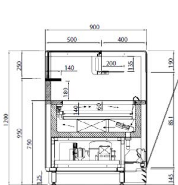
NEXT TOTAL Hauteur 1 200 mm
