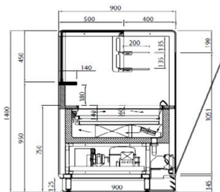
NEXT TOTAL Hauteur 1 400 mm
