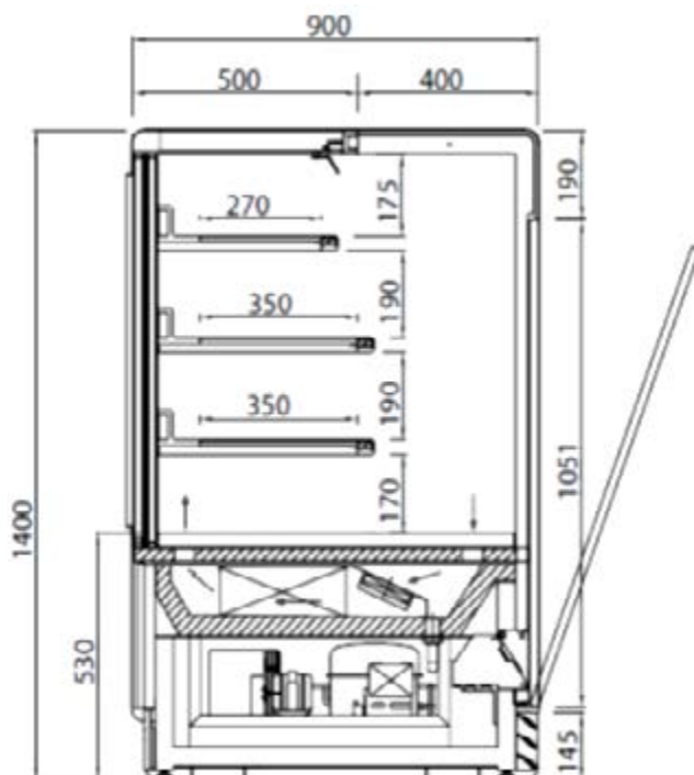
NEXT FULL Hauteur 1 400 mm
