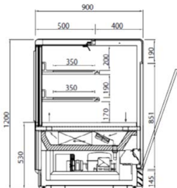
NEXT FULL Hauteur 1 200 mm
