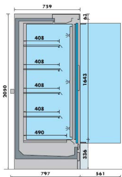
Versions à portes 750 - 2050
