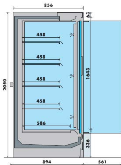
Versions à portes 850 - 2050
