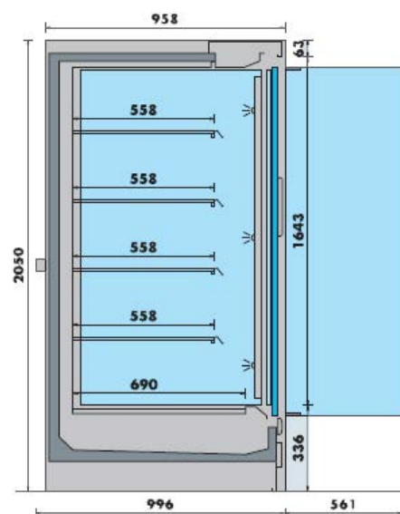
Versions à portes 950 - 2050
