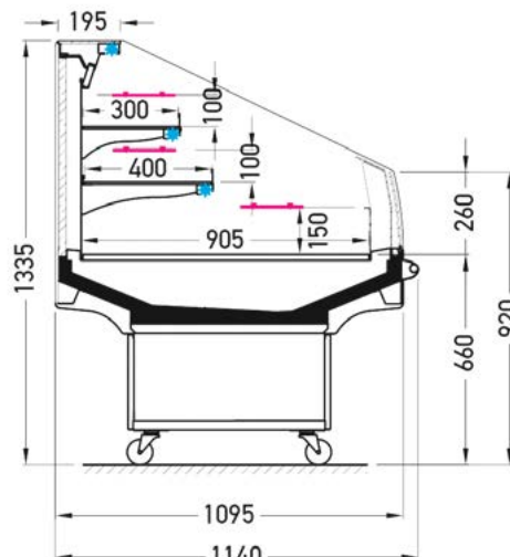
Version sans couvercle
