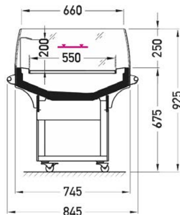
Version sans couvercle
