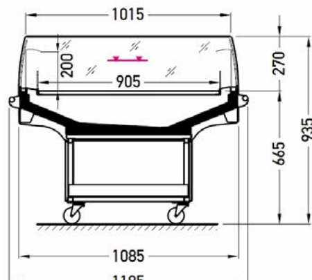
Version sans couvercle
