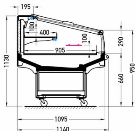
Version avec couvercle
