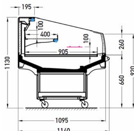
Version sans couvercle
