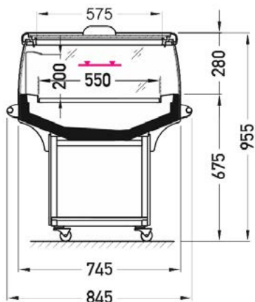
Version avec couvercle
