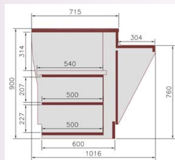
Coupe caisse PMR
