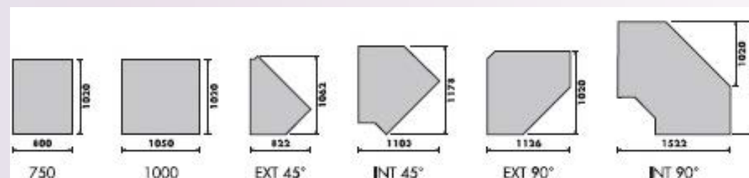
Coupe caisse standard
