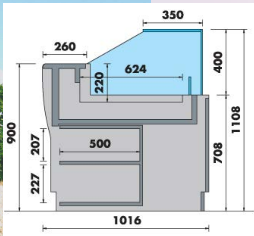
Coupe Version réfrigérée
