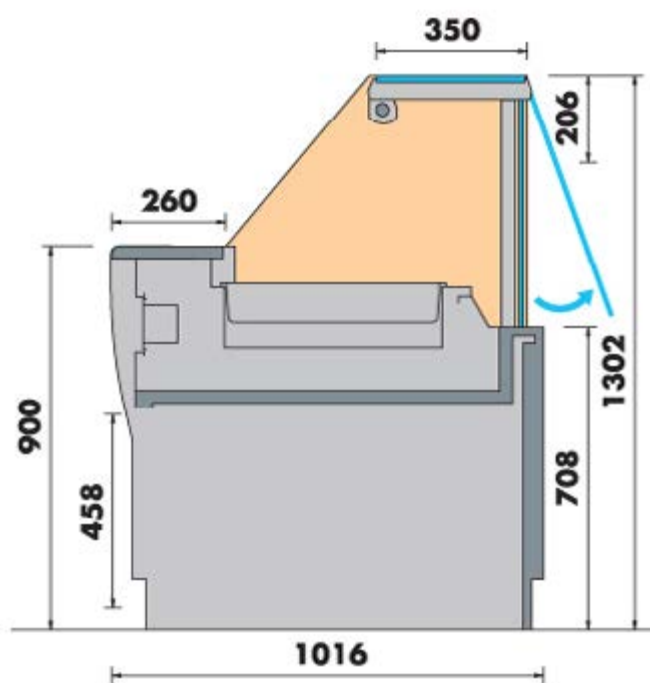
Version bain marie
