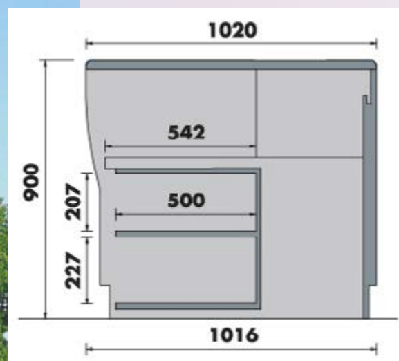
Coupe caisse standard
