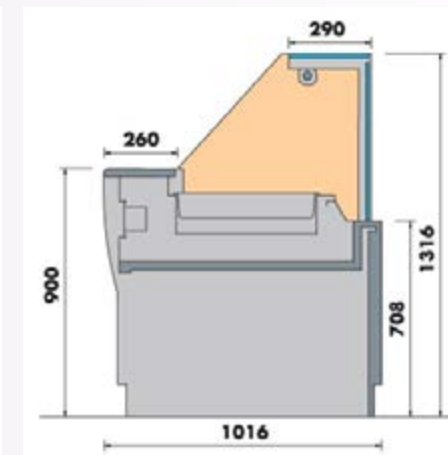
Version bain marie
