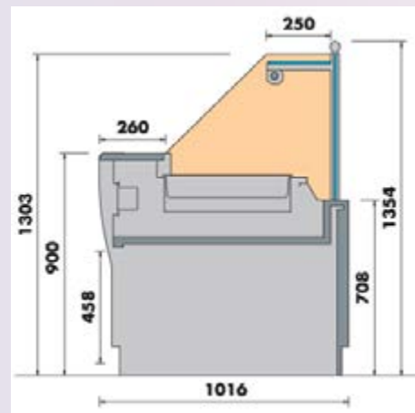
Version bain marie
