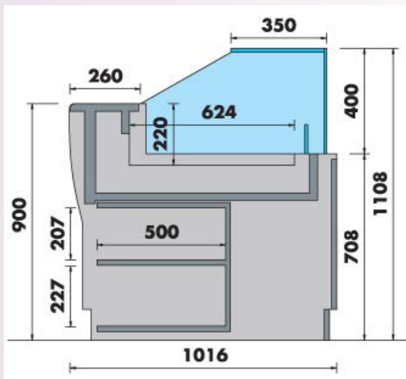
Coupe Version chocolat
